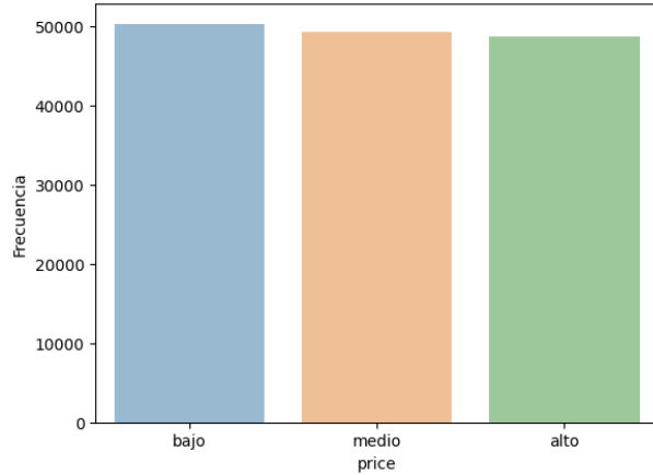
Igual frecuencia
