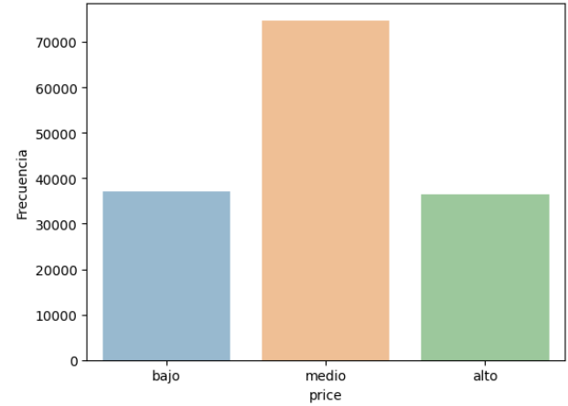
Cuartiles
